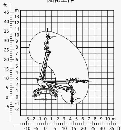
轨道轮工作
