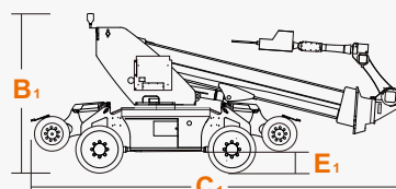
陆轮状态
